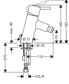
Talis S 32228000
