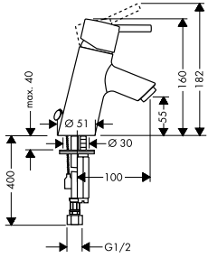
Talis S 32034000
