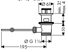
Talis S 32020000 / 32024000 / 32020003 / 32026000 / 32028000 / 32031000 / 32034000
