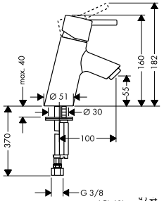
Talis S 32031000
