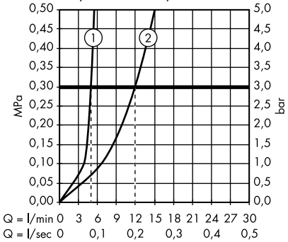
Talis S 32020000 / 32024000 / 32020003 / 32026000 / 32028000 / 32031000 / 32034000
